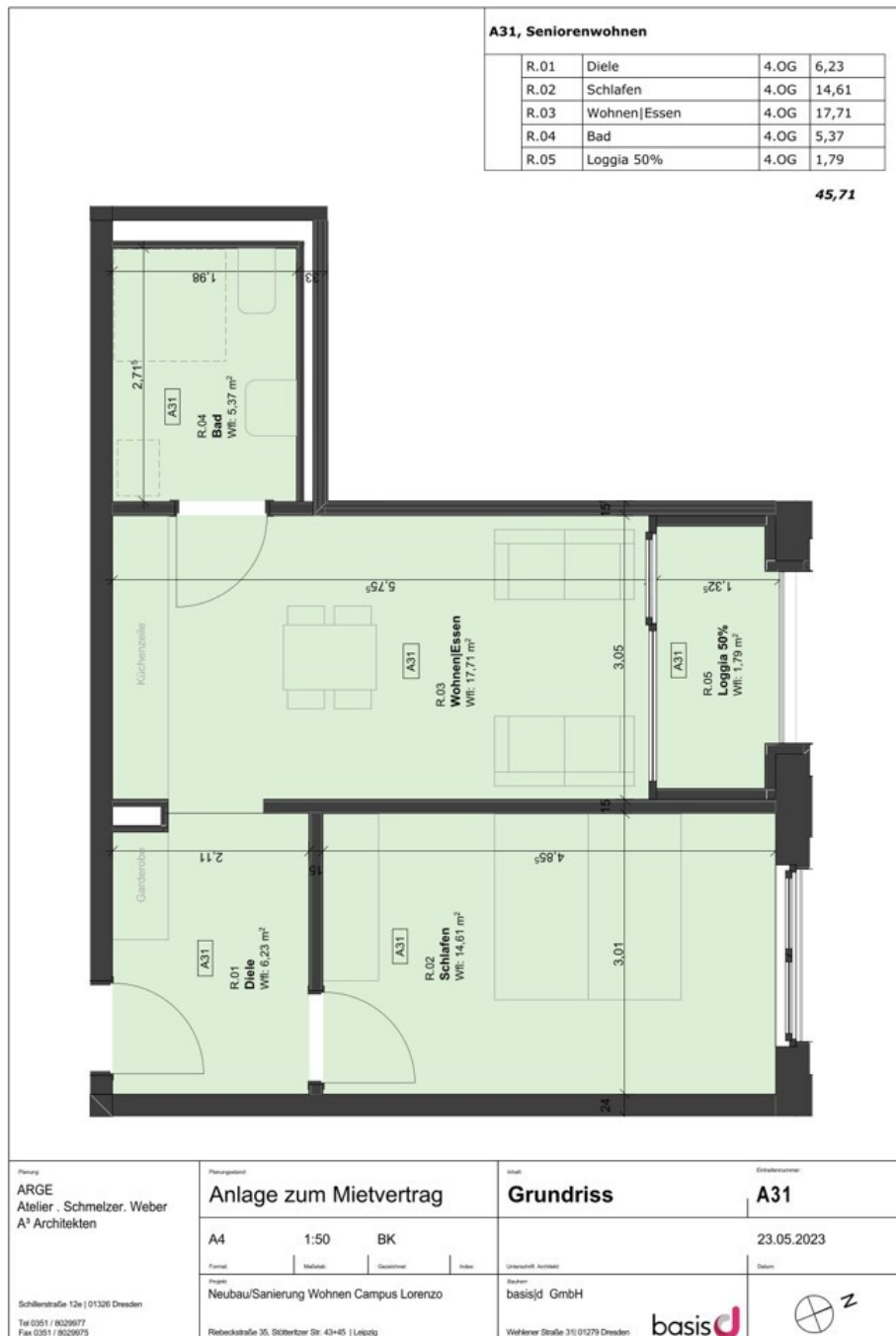
A31 - Seniorenwohnen mit Loggia - 4. OG
